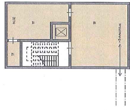
Grundriss UG
