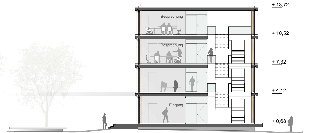
Schnitt M 1:200
