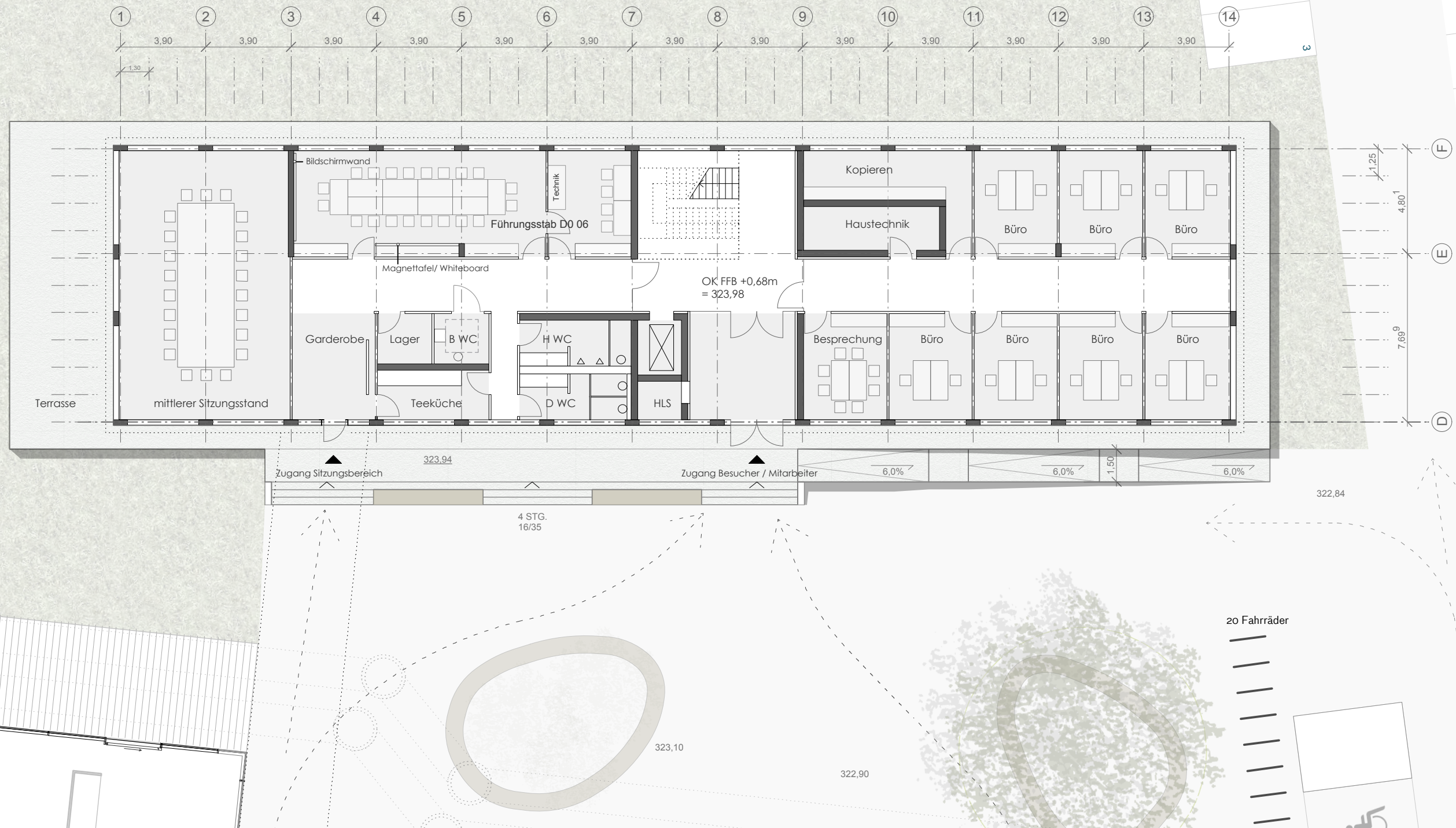
Grundriss Führungsstab Erdgeschoss M 1:200
