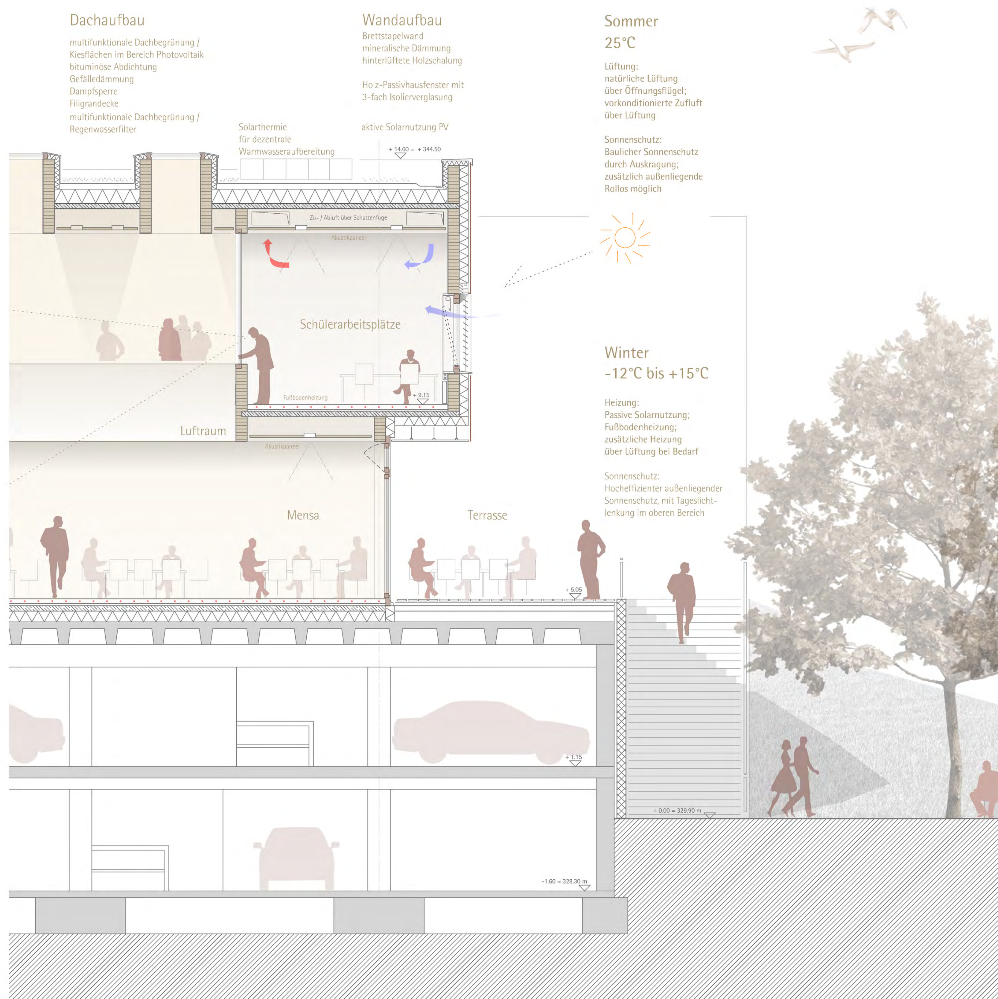
FASSADENSCHNITT M 1:50
