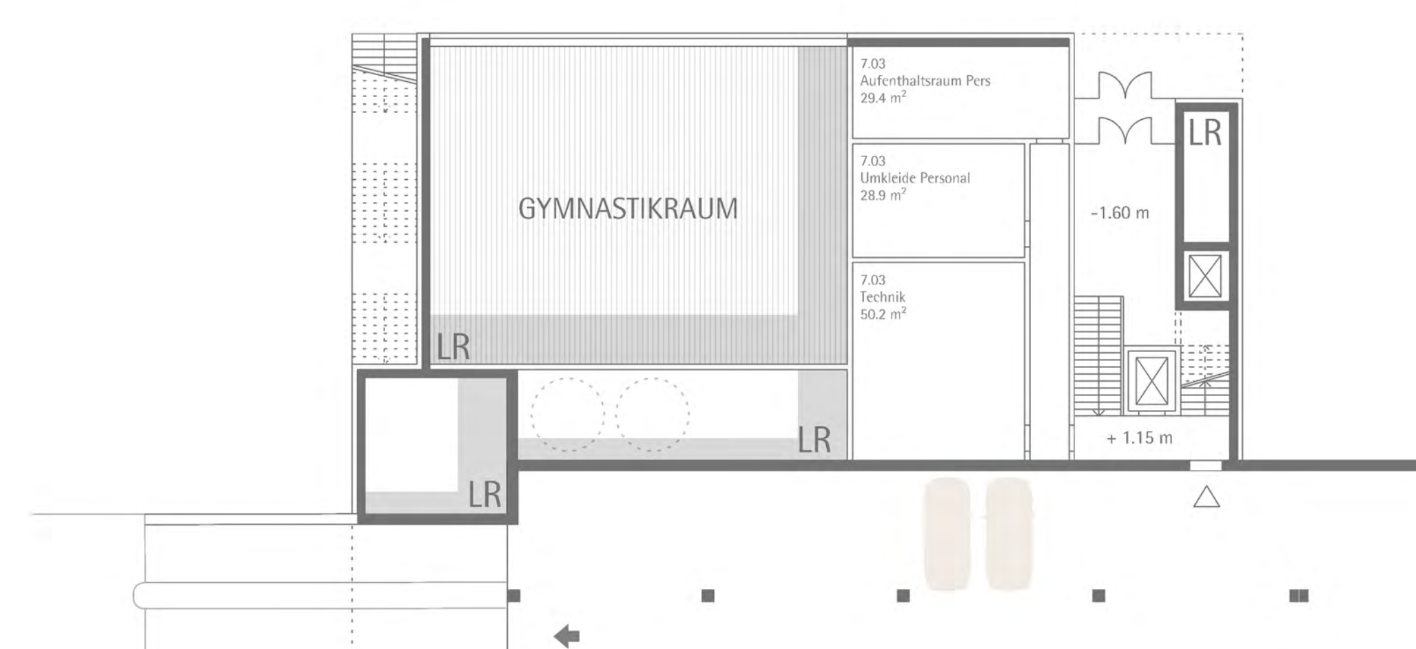
GRUNDRISS ZWISCHENGESCHOSS (TECHNIK) M 1:200
