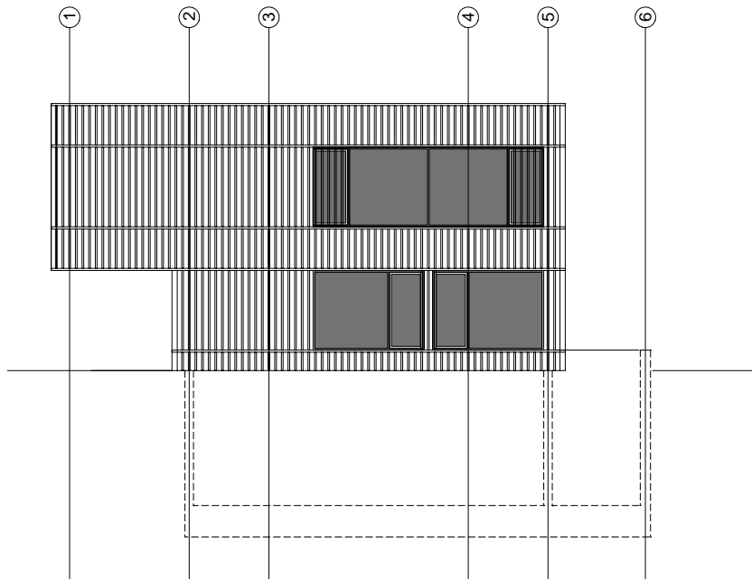
ANSICHT WEST
