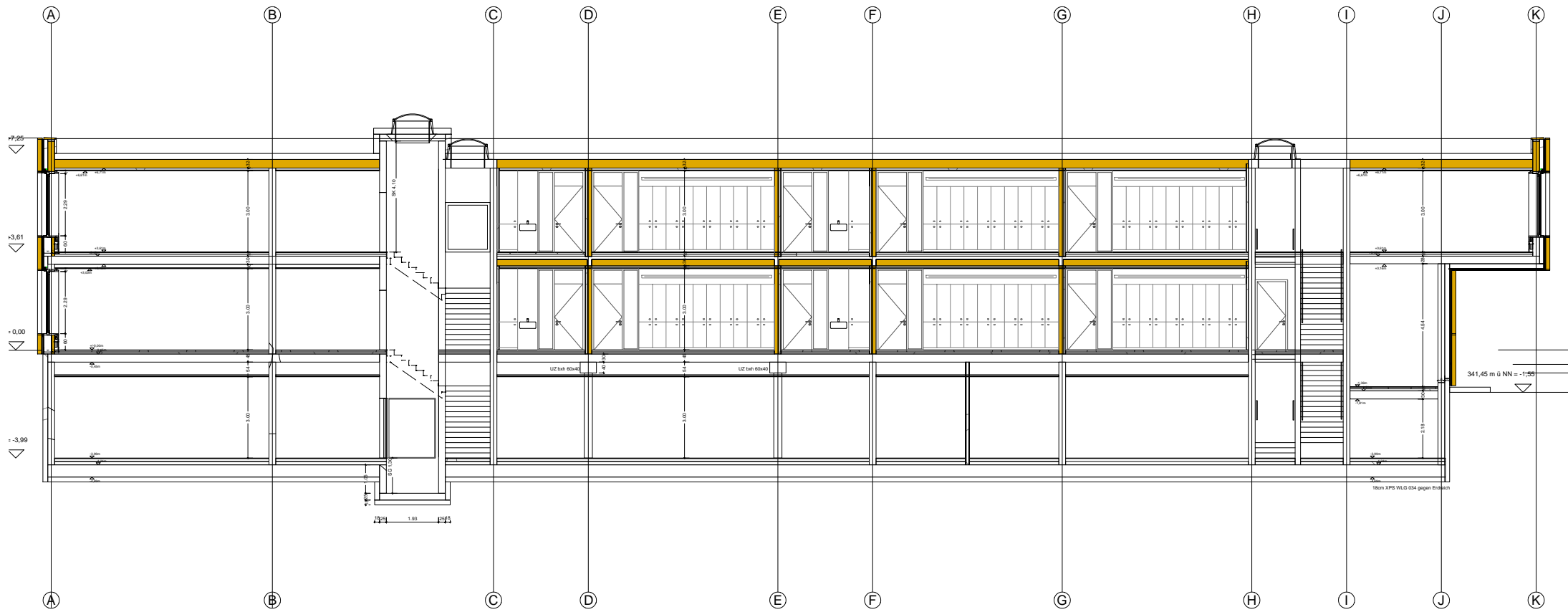
LÄNGSSCHNITT
