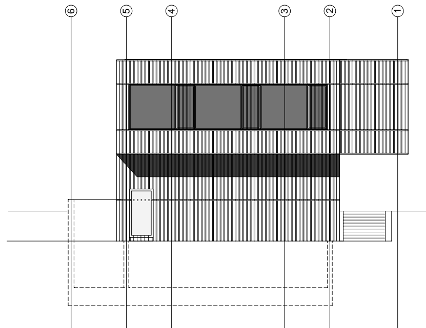
ANSICHT OST
