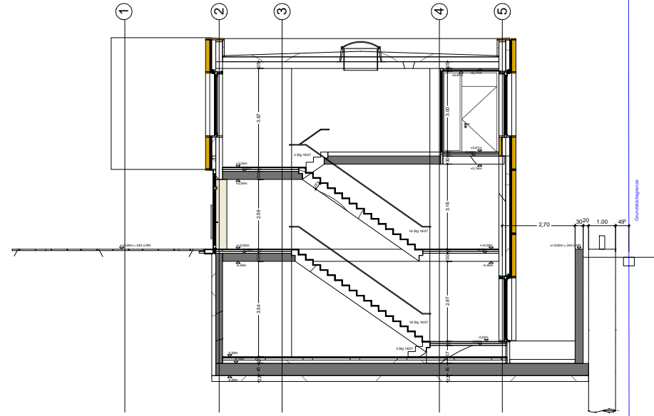
QUERSCHNITT 2
