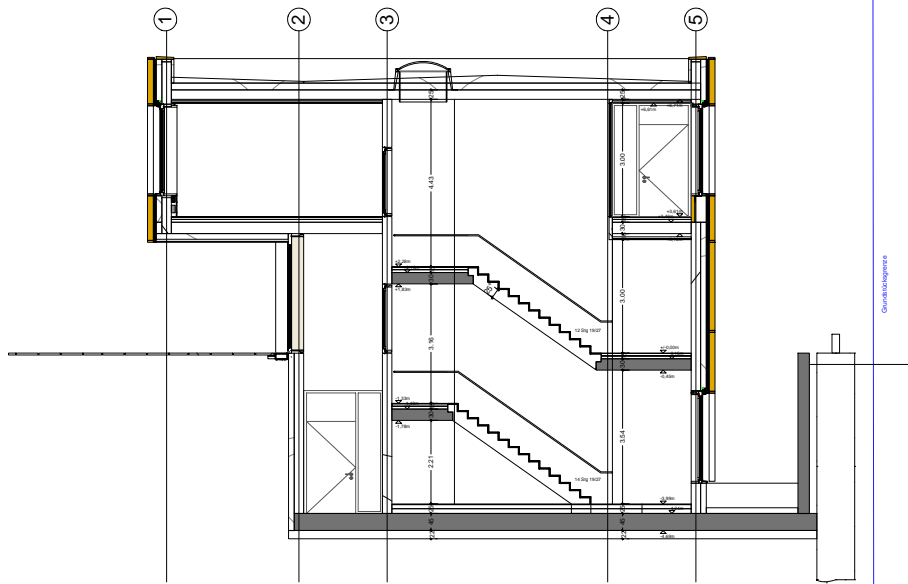
QUERSCHNITT 1
